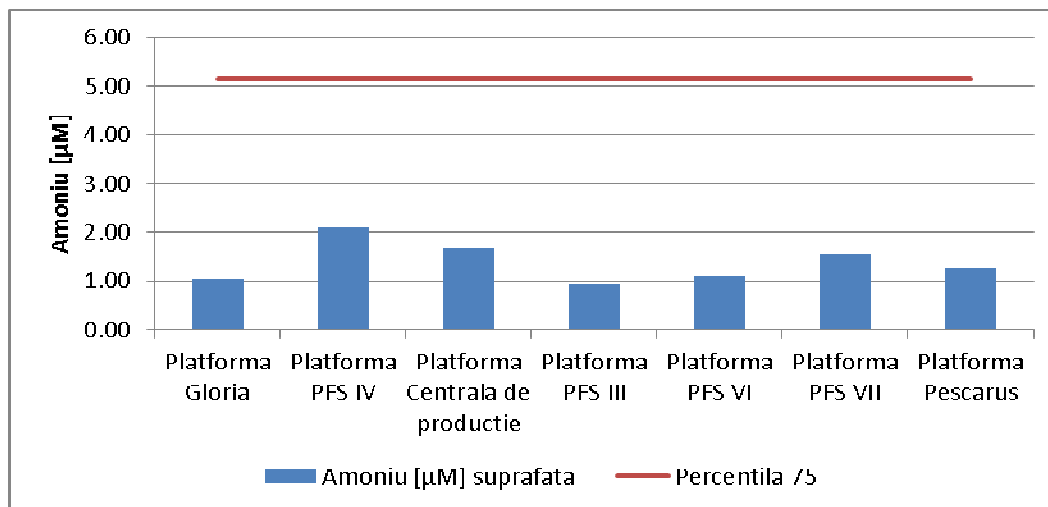
Fig.3.1.12a – Concentrațiile amoniului în apele marine de suprafață comparate cu percentila 75 a datelor istorice din zona de studiu
