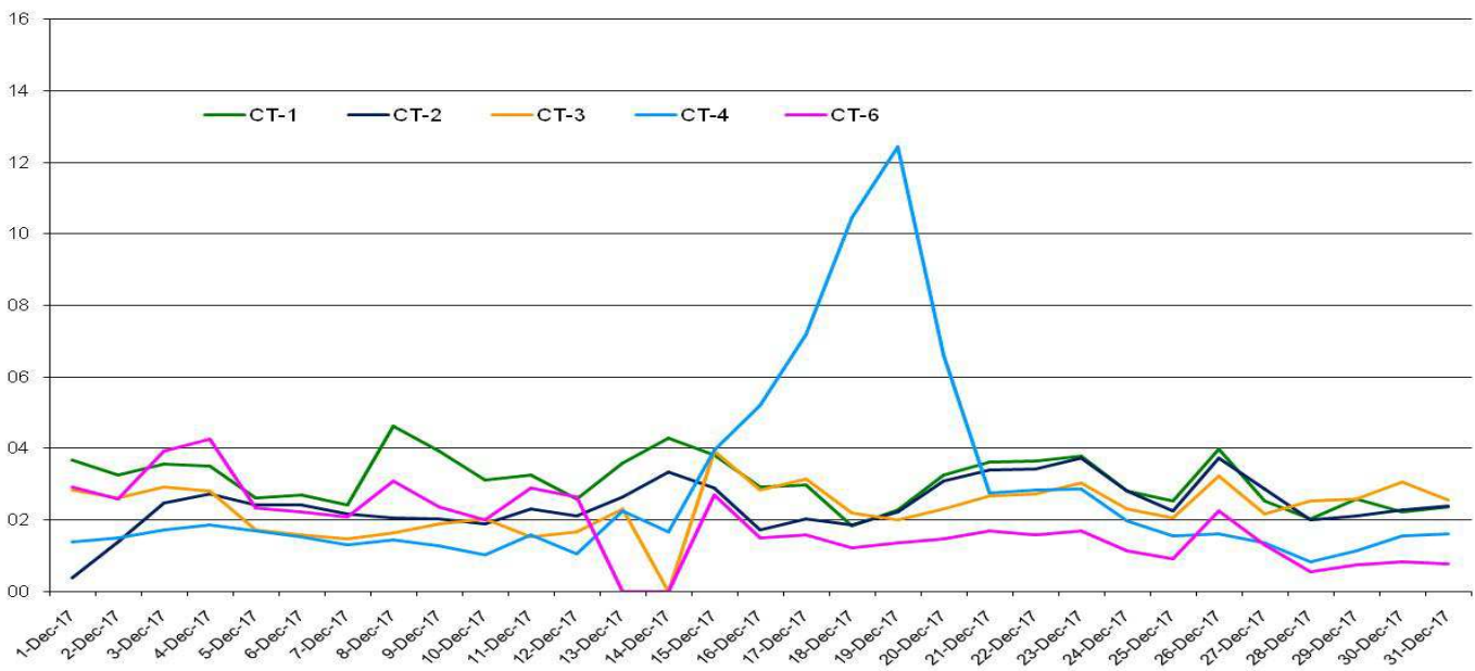
Benzen (ug/m3), perioada: 01 Decemb 2017- 31 Decemb 2017 - Date validate
