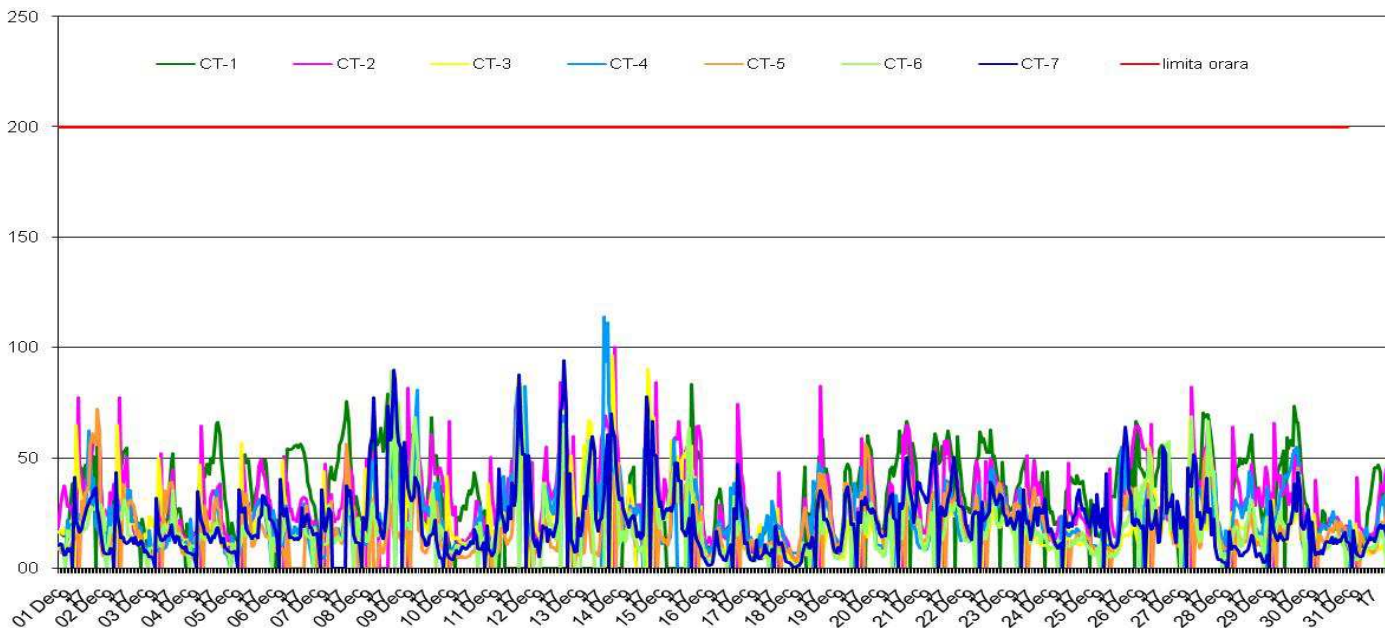
NO2 (ug/m3), perioada: 01 Decemb 2017-31 Decemb 2017 - Date validate
