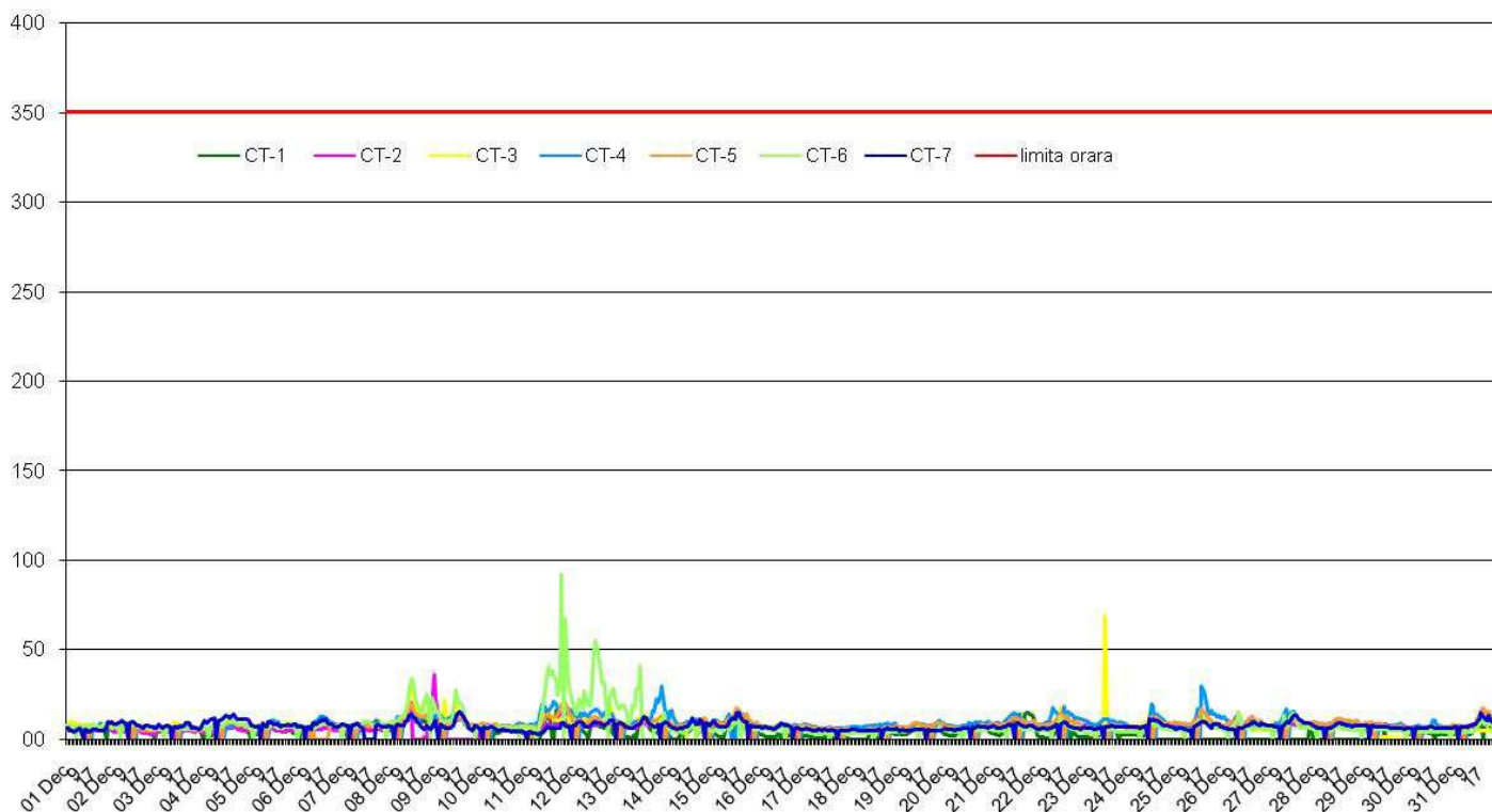
SO 2 (ug/m3), perioada: 01 Decemb 2017-31 Decemb 2017 - Date validate
