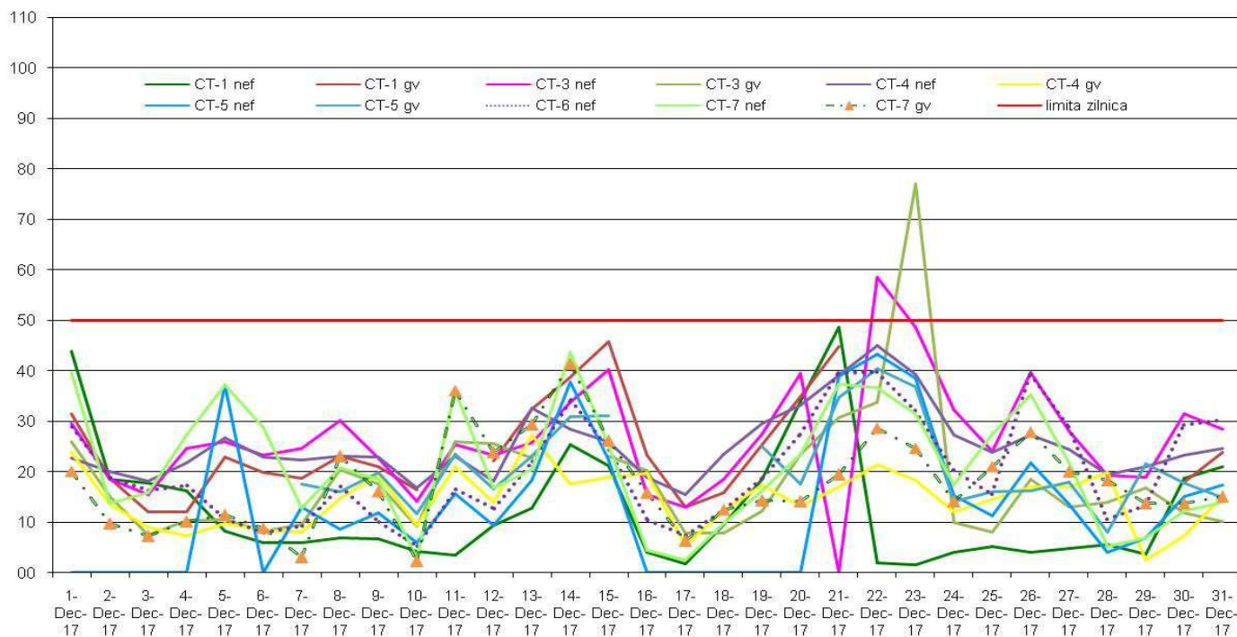
PM10 nef si PM10 gv (ug/m3), perioada: 01 Decemb 2017-31 Decemb 2017 - Date validate
