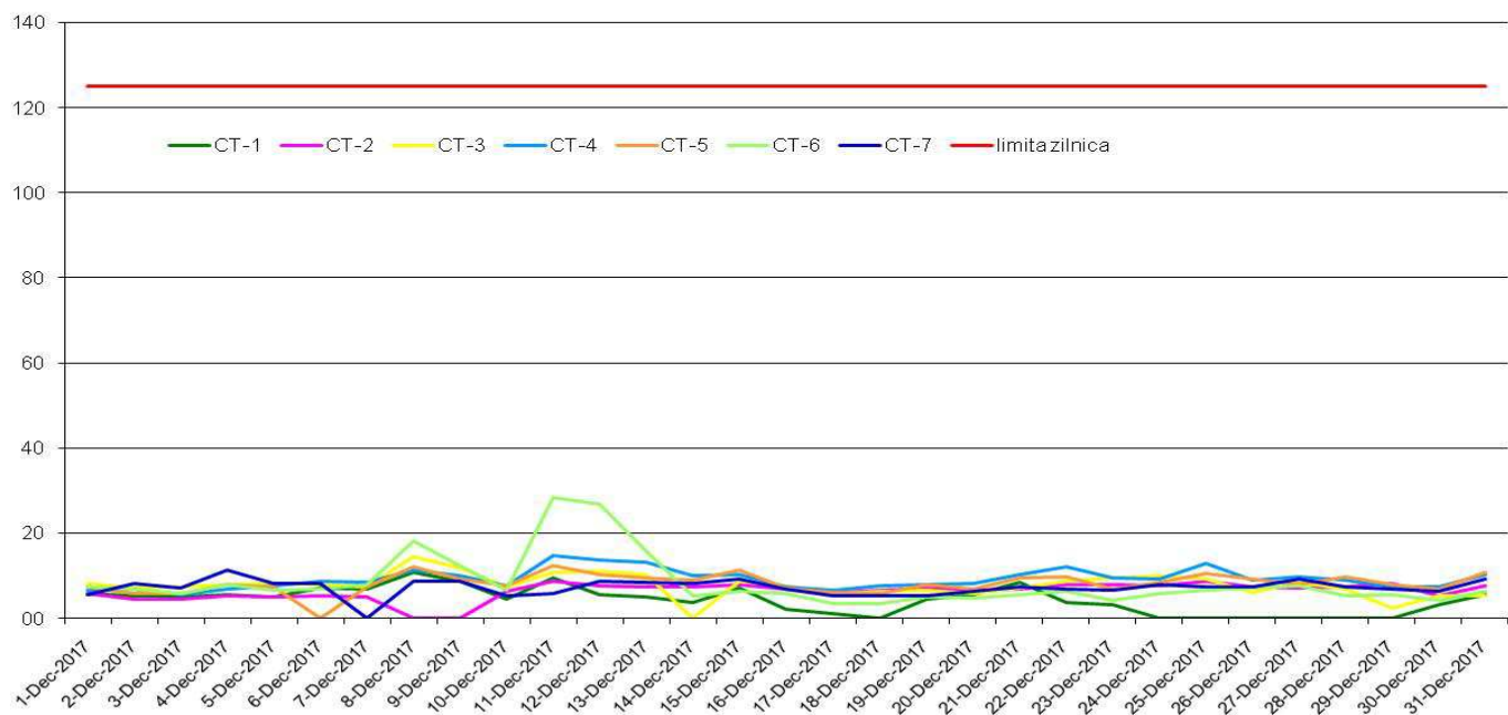
SO2 (ug/m3), perioada: 01 Decemb 2017-31 Decemb 2017 - Date validate
