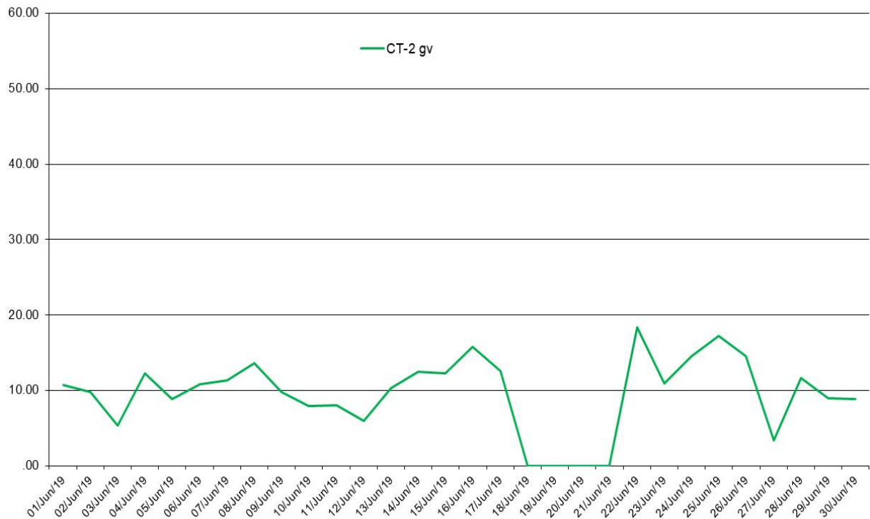
PM2.5 gv (ug/m3), perioada: 01 - 30 Iunie 2019 - Date validate
