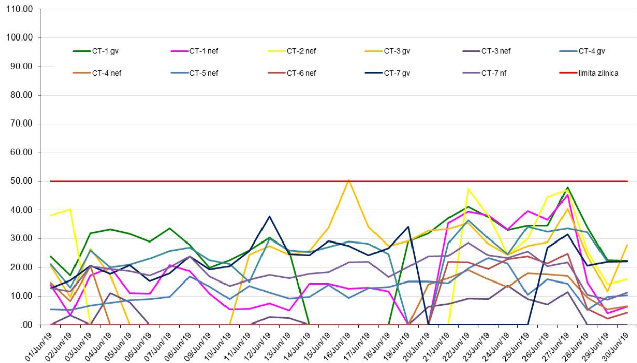
PM10 nef si PM10 gv (ug/m3), perioada: 01 - 30 Iunie 2019 - Date validate
