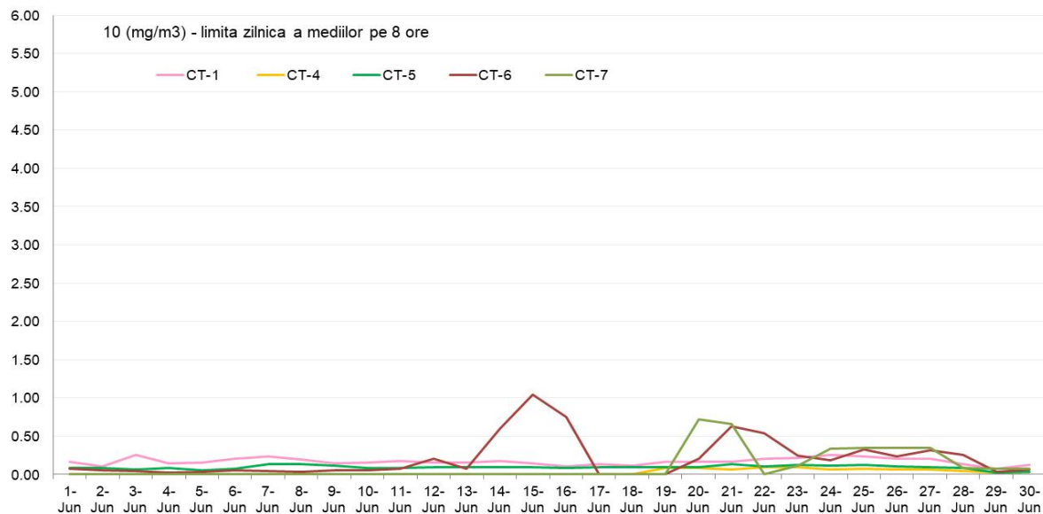
CO (mg/m3) - maximul zilnic medie mobila perioada: 01 Iunie - 30 Iunie 2019 - date validate
