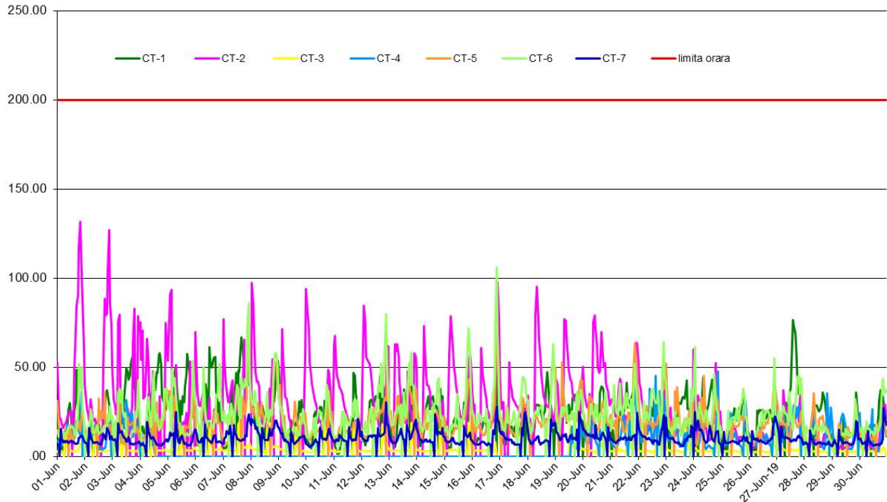
NO2 (ug/m3), perioada: 01 Iunie 2019 - 30 Iunie 2019 - Date validate
