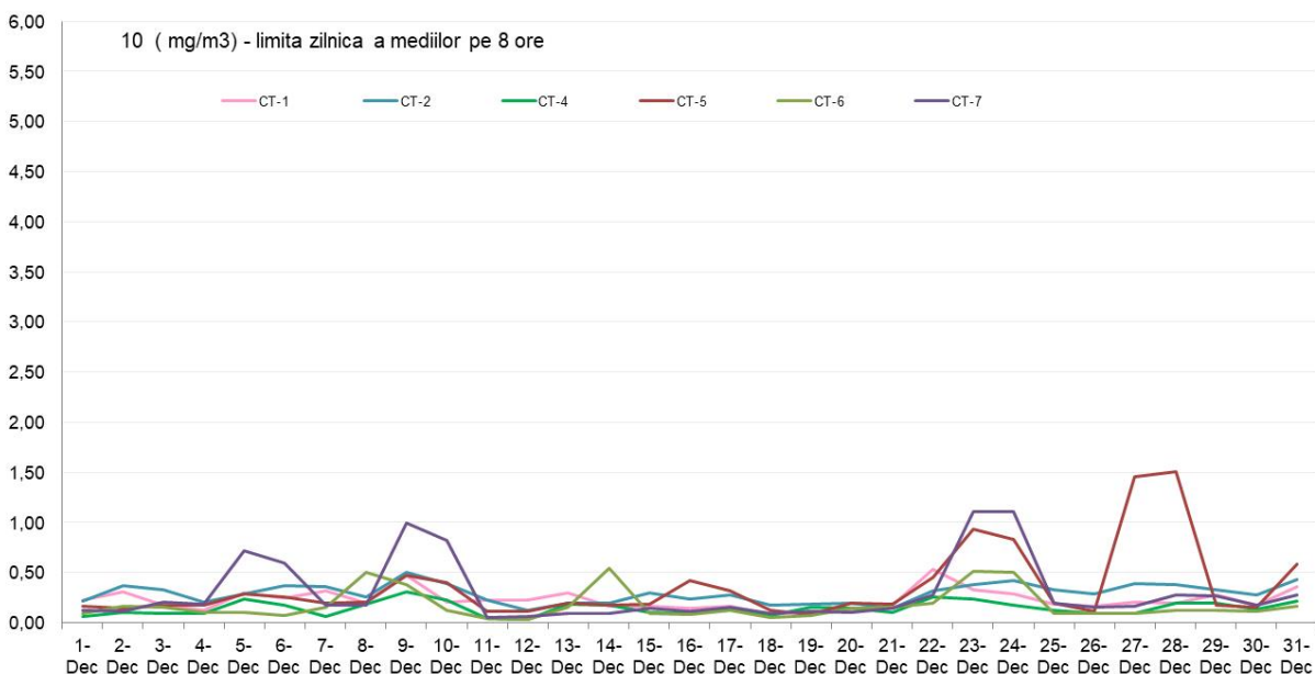
CO (mg/m3) - maximul zilnic medie mobila perioada: 01 - 31 Decembrie 2021 - date validate
