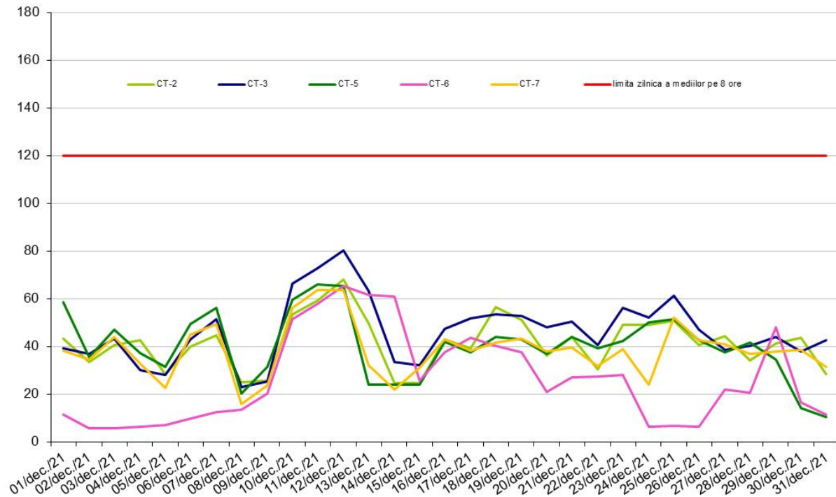
O 3 (mg/m 3 ) - maximul zilnic medie mobila perioada: 01 - 31 Decembrie 2021 - date validate
