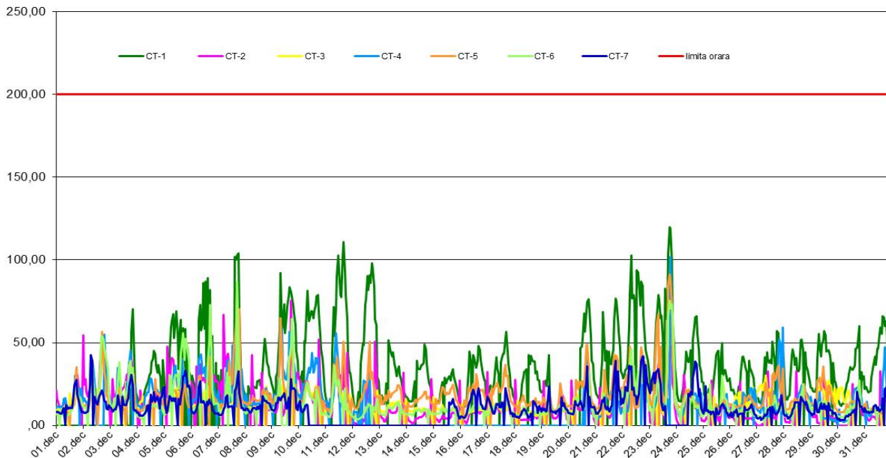
NO2 (ug/m3), perioada: 01 - 31 Decembrie 2021 - Date validate
