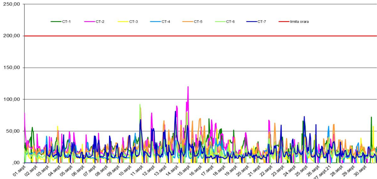
NO 2 (ug/m3), perioada: 01 - 30 Septembrie 2021 - Date validate
