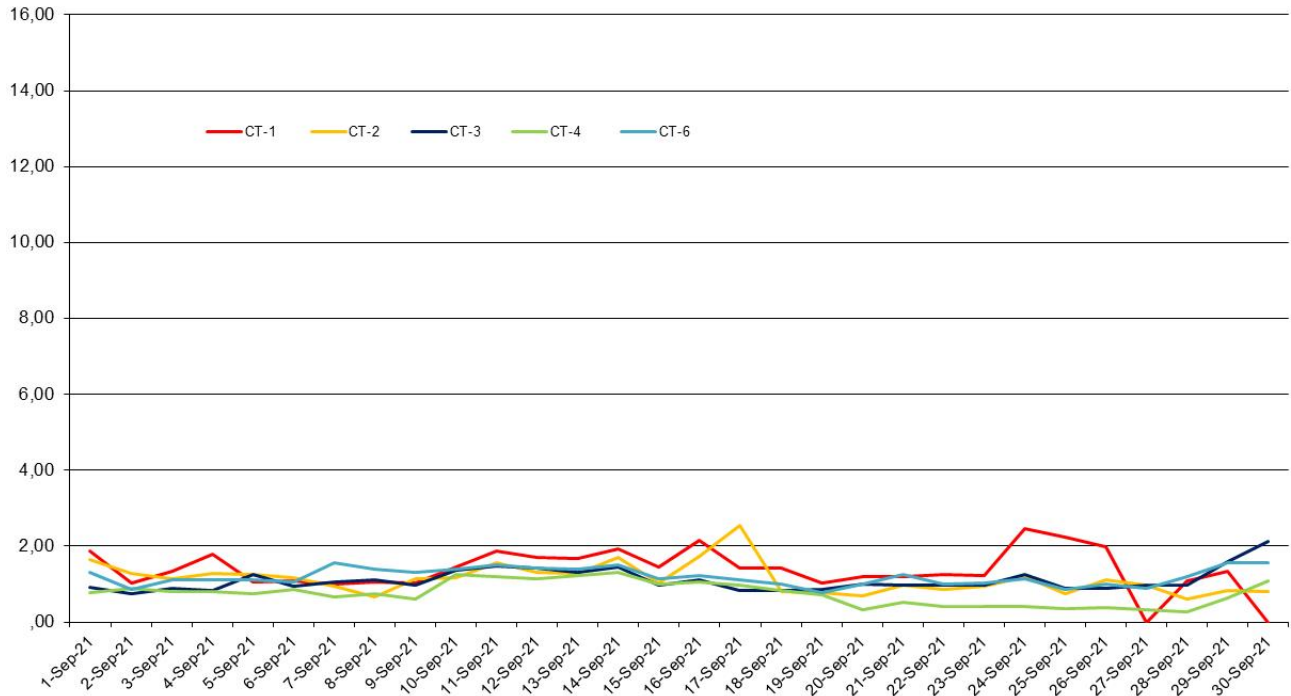
Benzen (ug/m3), perioada: 01 - 30 Septembrie 2021 - Date validate
