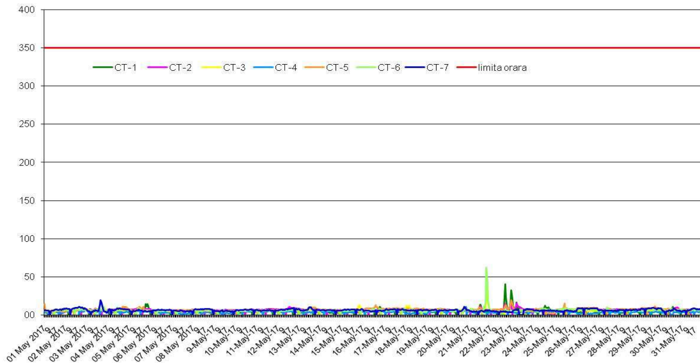
SO 2 (ug/m3), perioada: 01 Mai 2017-31 Mai 2017 - Date validate
