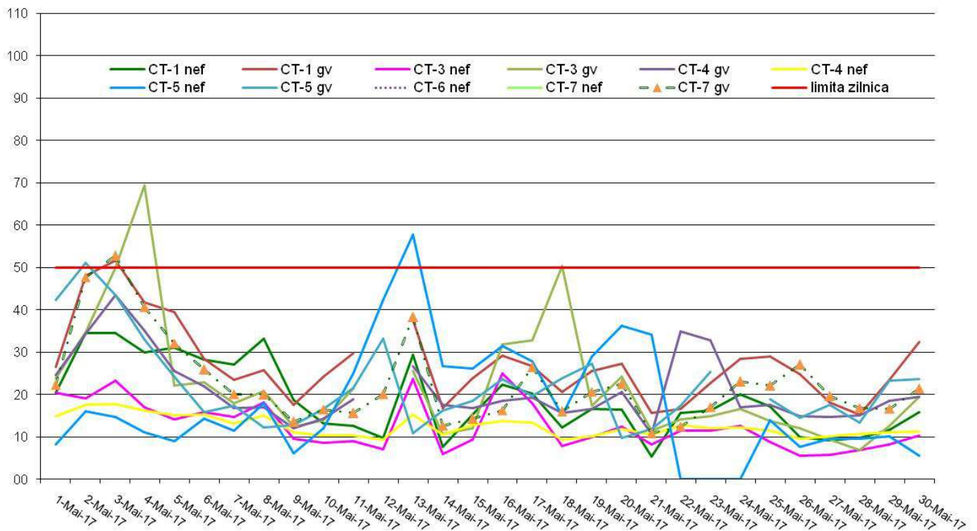
PM10 nef si PM10 gv (ug/m3), perioada: 01 Mai 2017-31 Mai 2017 - Date validate
