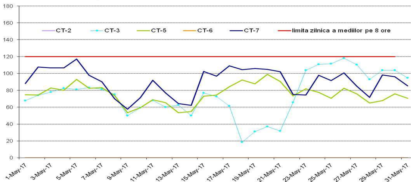
O 3 (mg/m 3 ) - maximul zilnic medie mobila perioada: 01 Mai - 31 Mai 2017 - date validate
