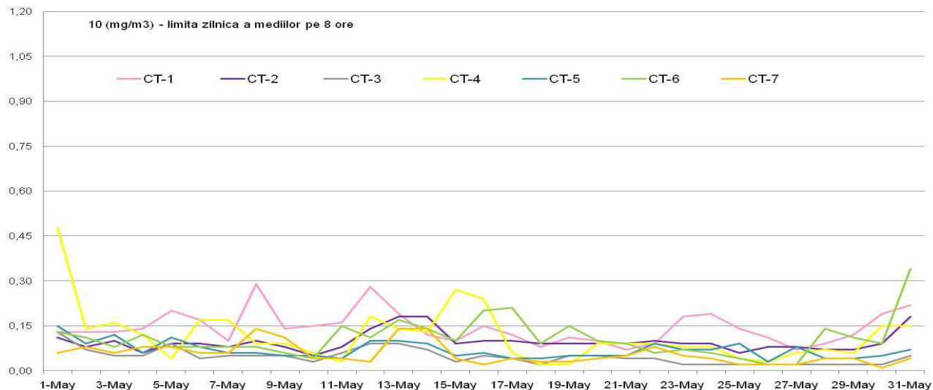
CO (mg/m 3 ) - maximul zilnic medie mobila perioada: 01 Mai - 31 Mai 2017 - date validate
