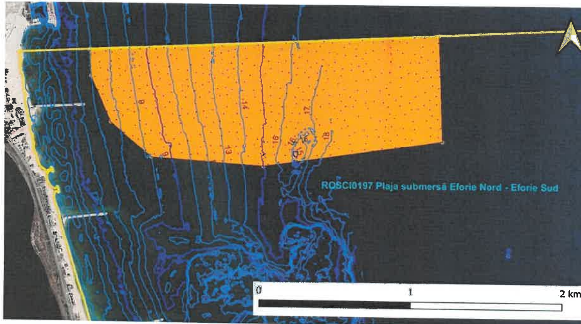
Figură 4 poligonul evidențiat cu portocaliu reprezintă zona de amplasare a structurilor dure de tip recifi artificiali delimitată preliminar la etapa de SF.
