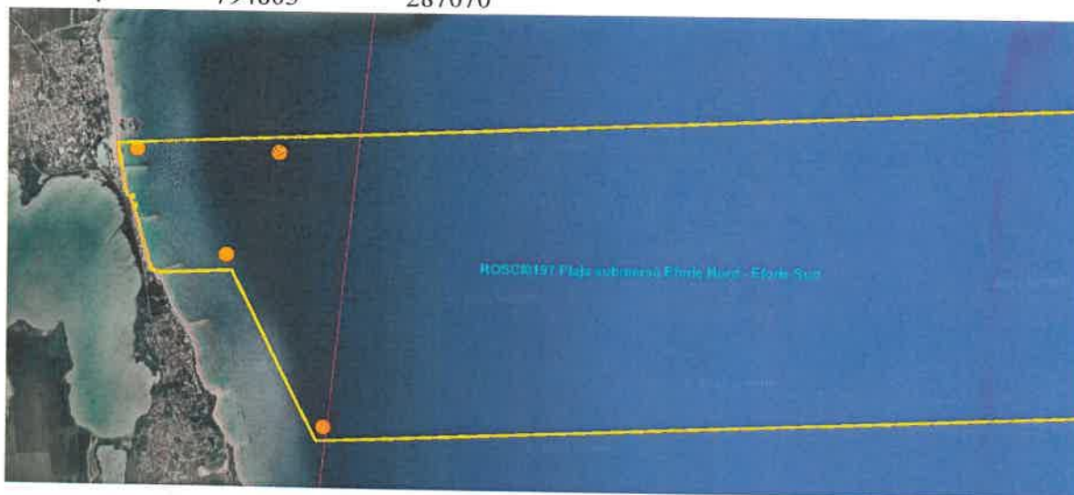
Figură 5 Cele 4 puncte evidențiate cu portocaliu indică zona de amplasare a capcanelor de sedimente stabilite la etapa de SF.
