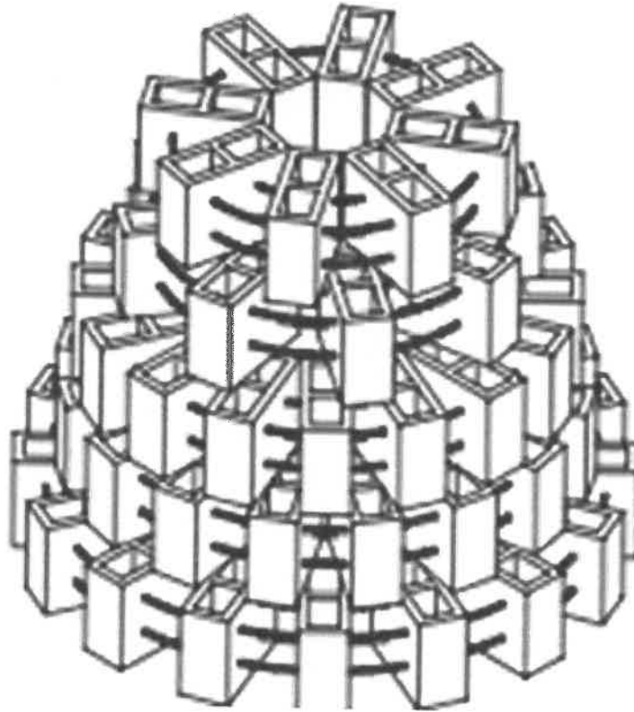
Figură 1 Schema constructivă a unui recif artificial de tip 1
