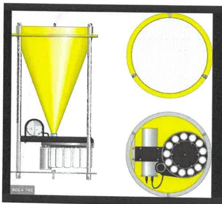
Figură 3 Schema constructivă a capcanei de sediment
