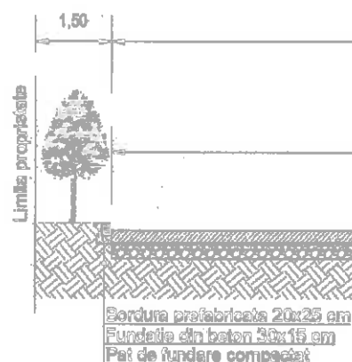
fig.2 Detaliu alcătuire
