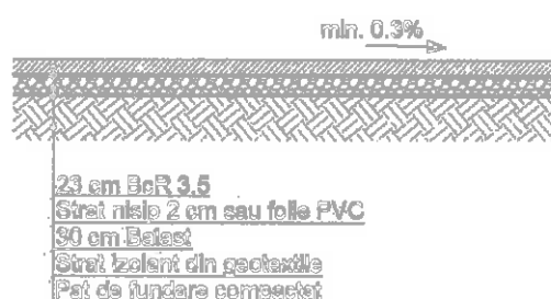
fig.1 Detaliu alcătuire
