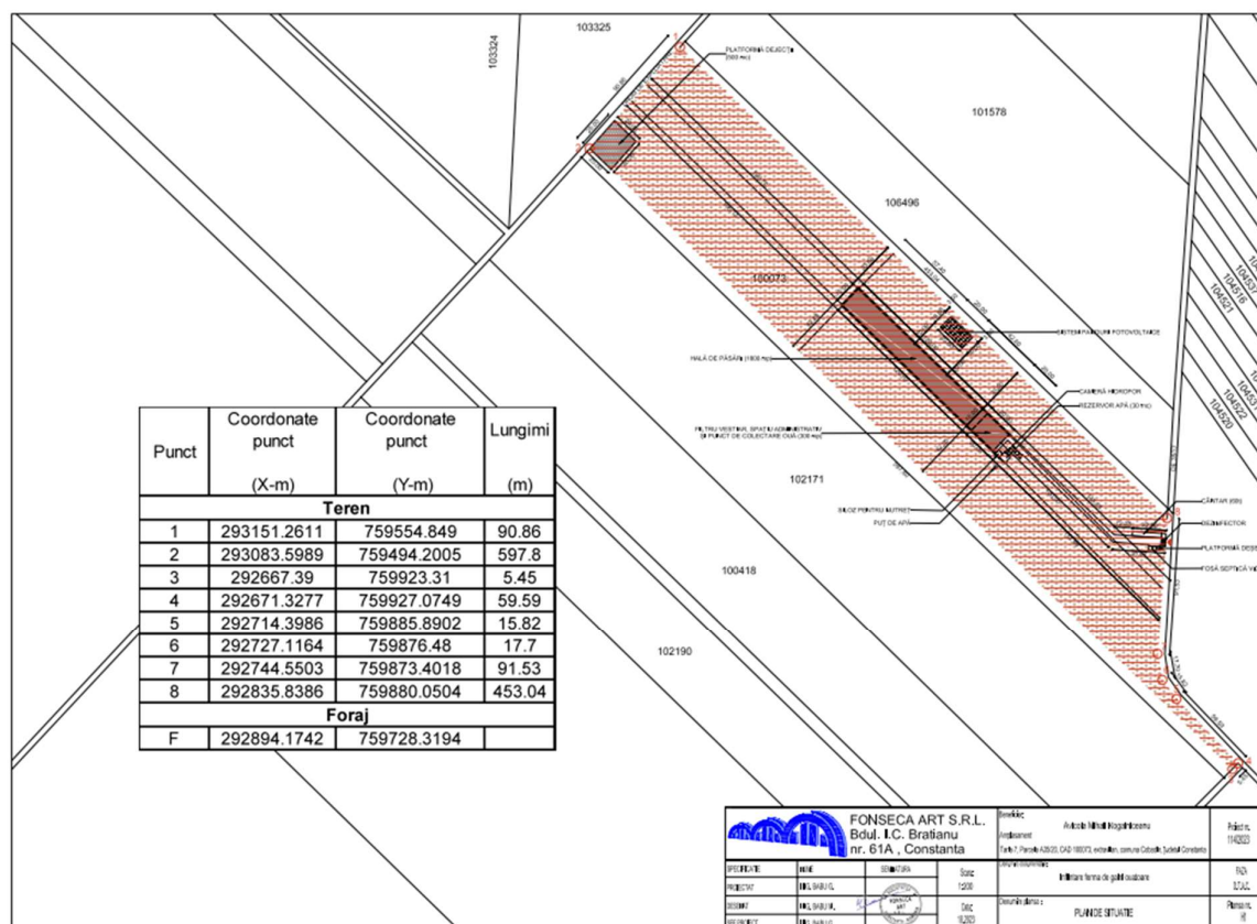
Fig.1 – Plan de situatie ferma pentru gaini ouatoare
