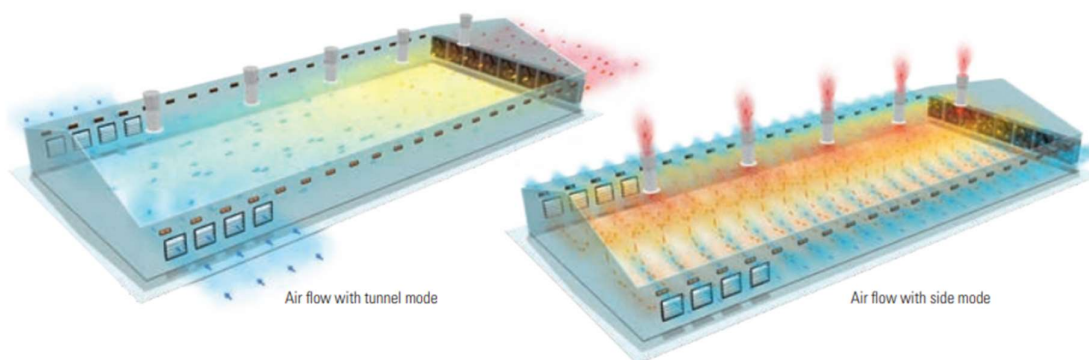
Fig. 10 – Sistem de ventilatie
