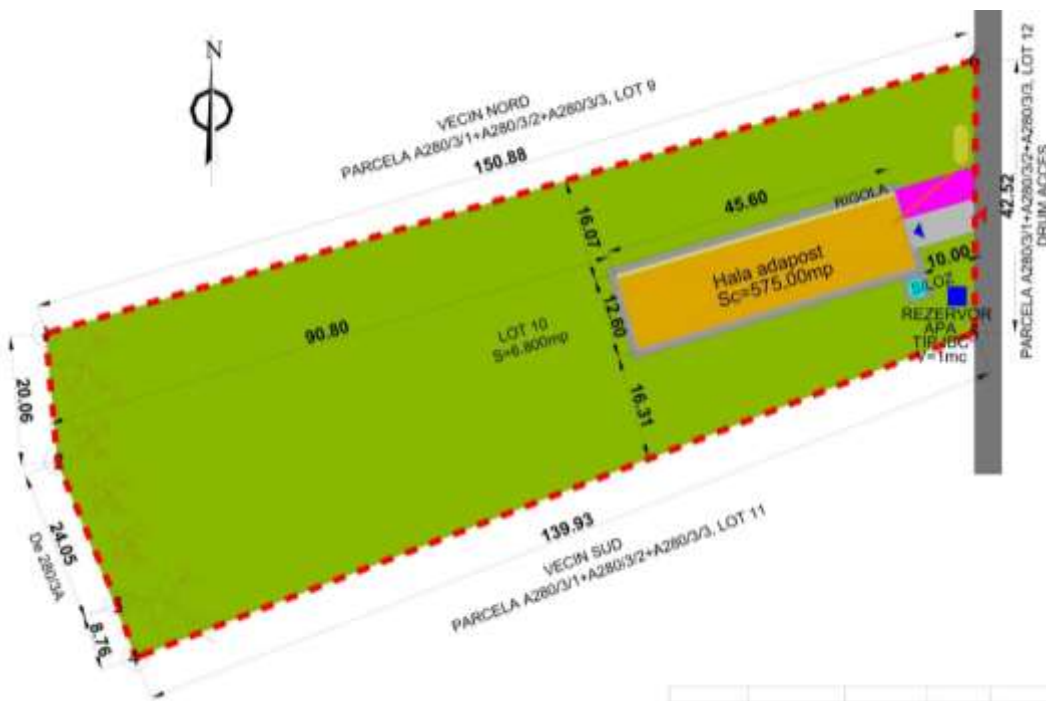
Figura 2- Plan de situatie Ferma 8 Farm Nutrition SRL
